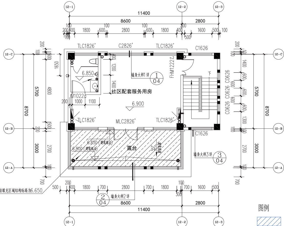
三层平面图
