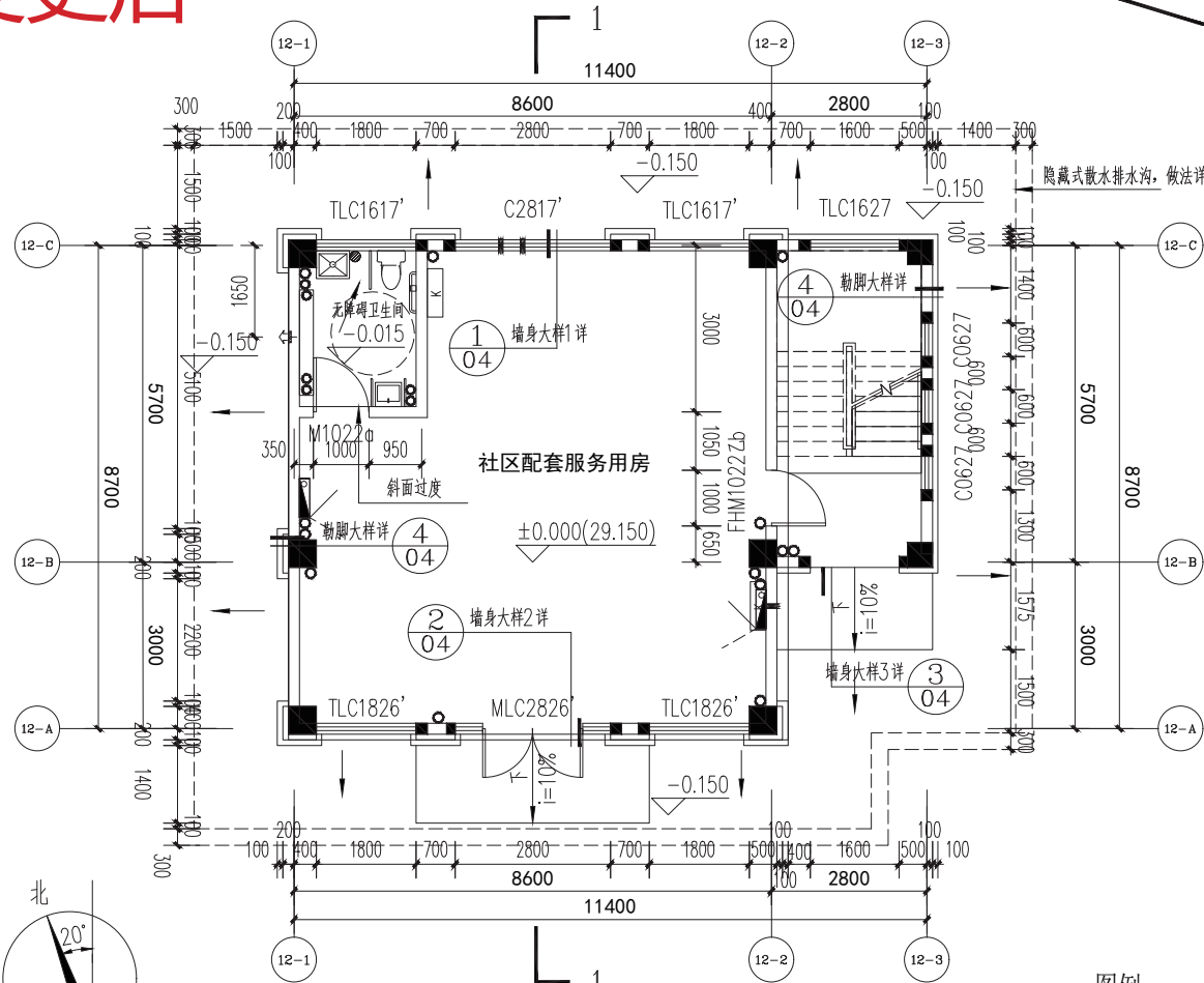
一层平面图
