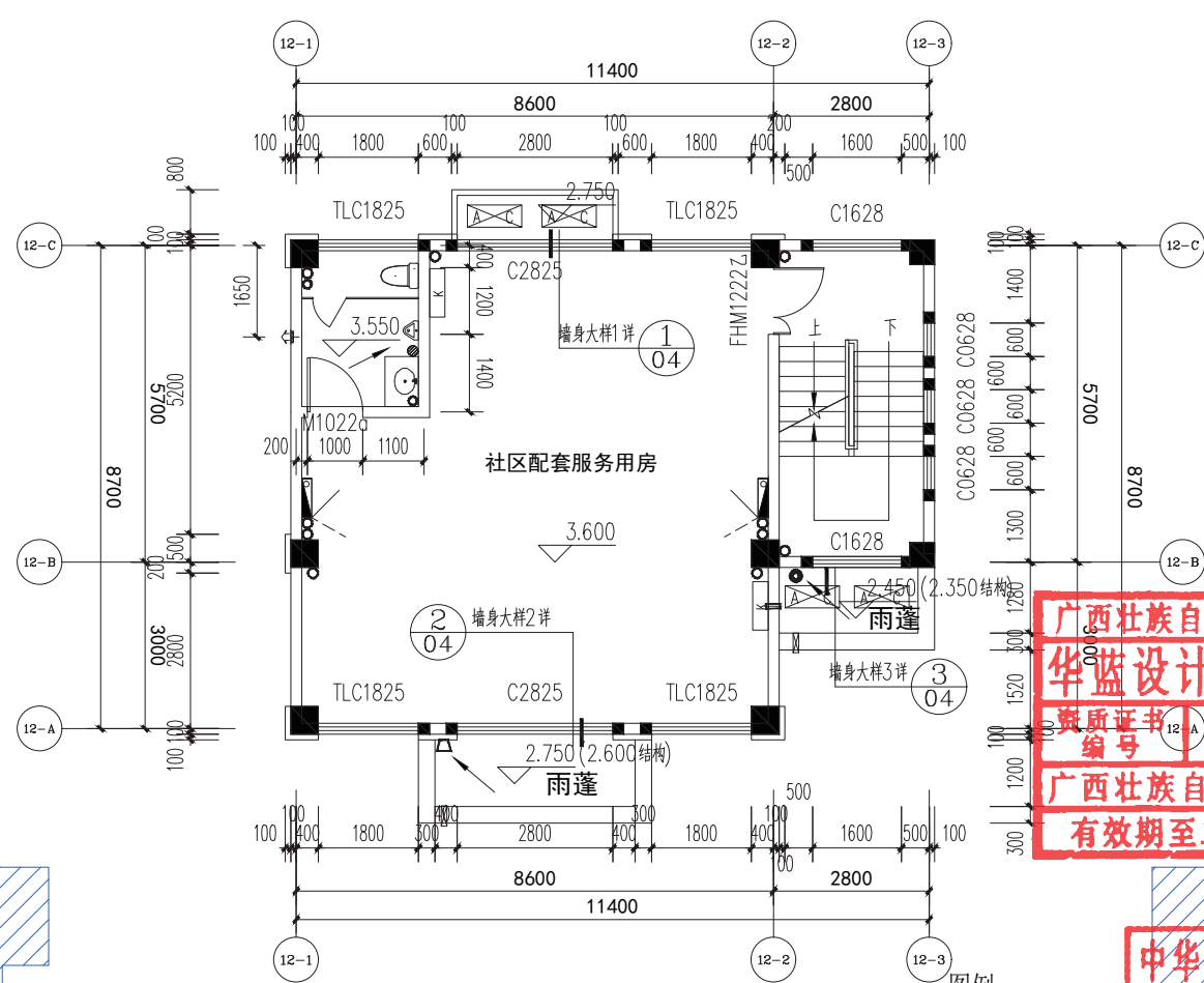
二层平面图
