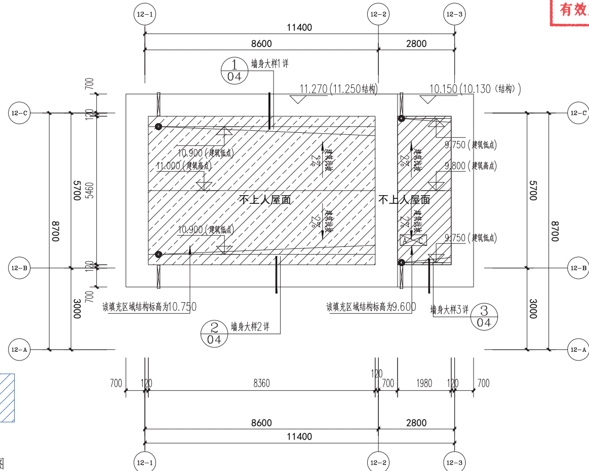
屋面层平面图
